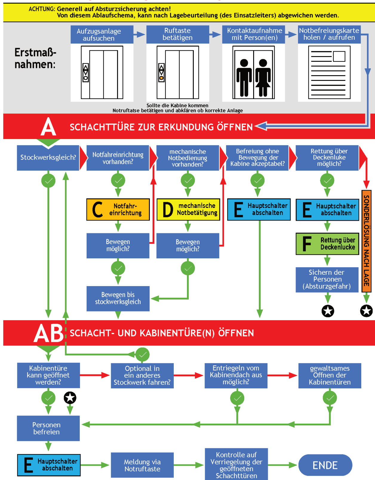
Abbildung 1: Notbefreiungsablaufdiagramm (Christopher Miksch)
