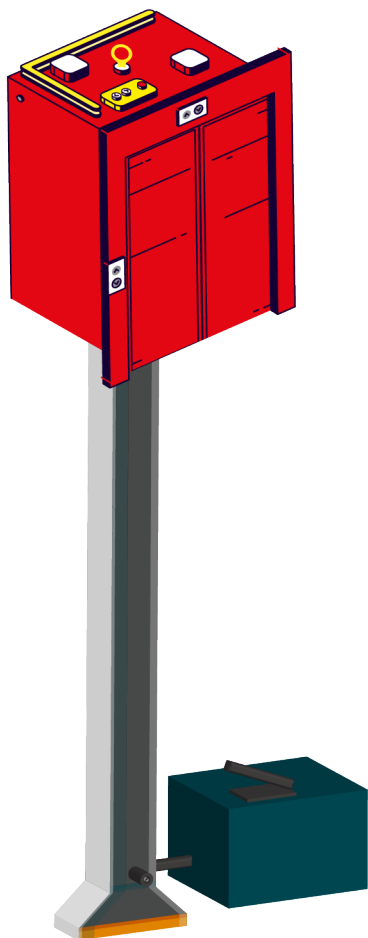
Abbildung 3: direkter hydraulischer Aufzug (R. Berger | FEUERWEHR.AT)
